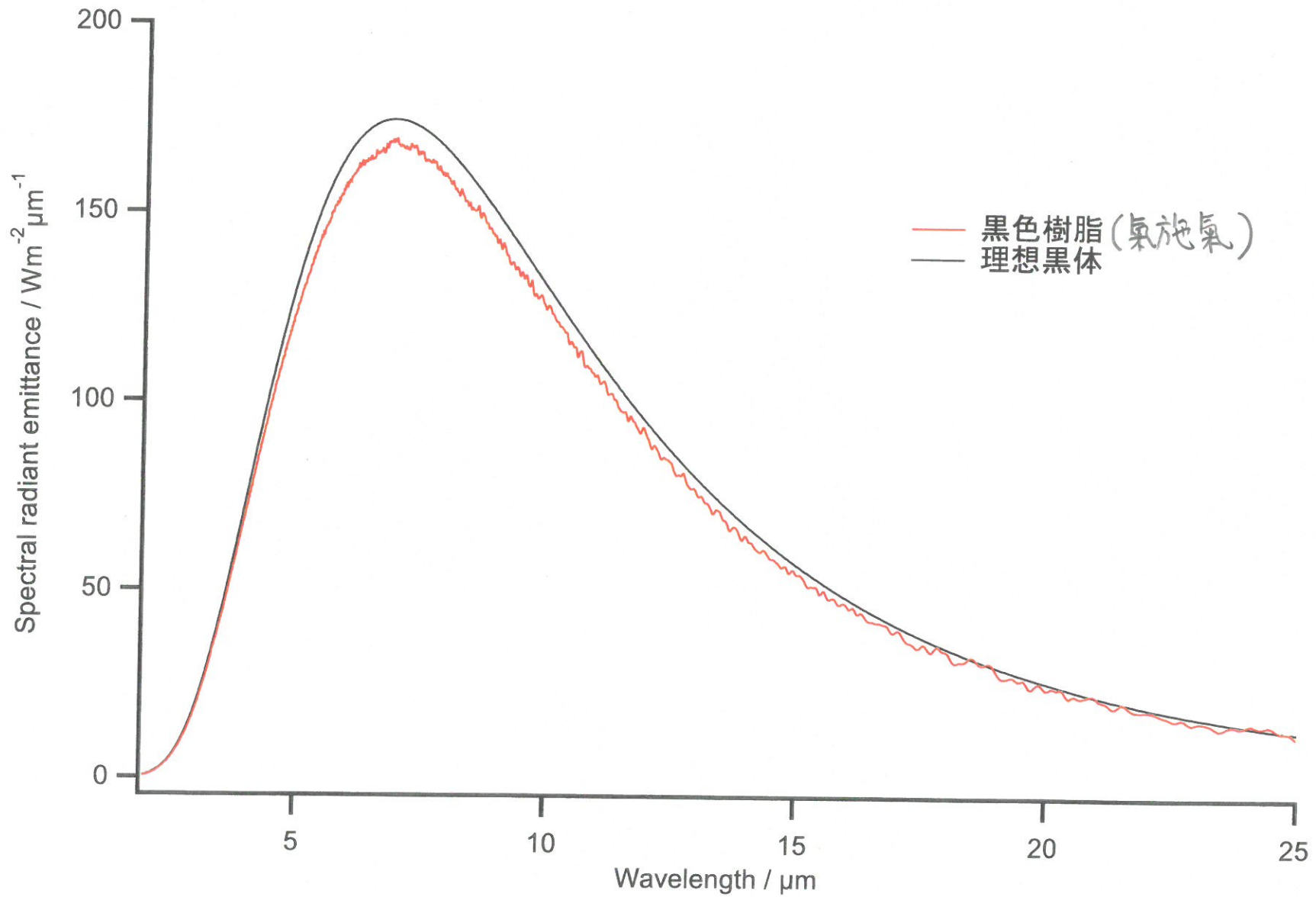
図3 150°Cにおける黒色樹脂と理想黒体の分光放射発散度 (2~25ミクロン) n=2回測定の平均値を表示
